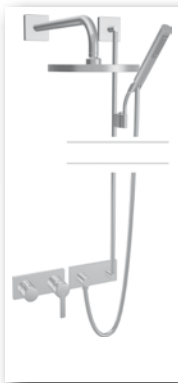
HANSAMATRIX Opbouwpakket 03 ééngreepsmengkraan, DN 15 (1/2")* 4487 2030 verchromd past bij HANSARONDA met glijstangset met HANSARAIN hoofddouche, DN 15
